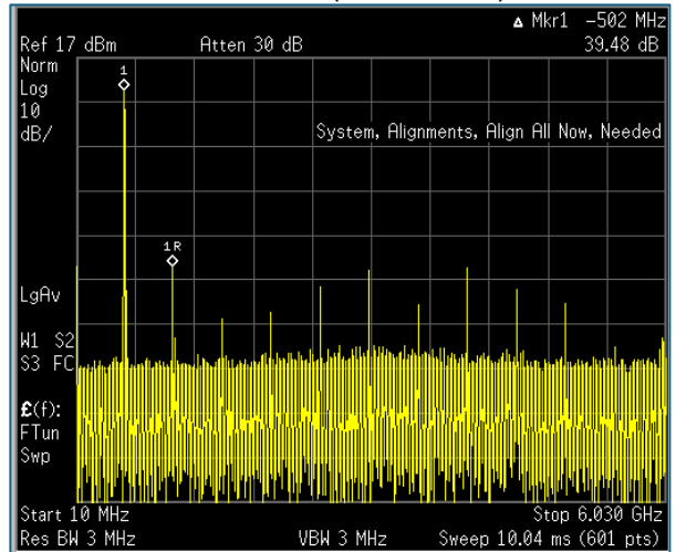
Harmonics (-34.78 dBc)
